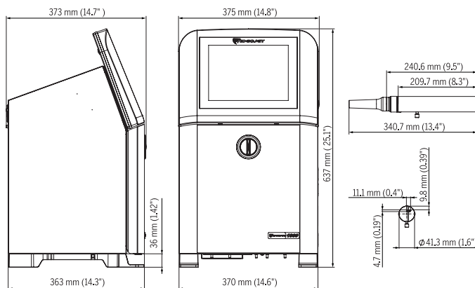
Las dimensiones mostradas se corresponden con el modelo IP66
